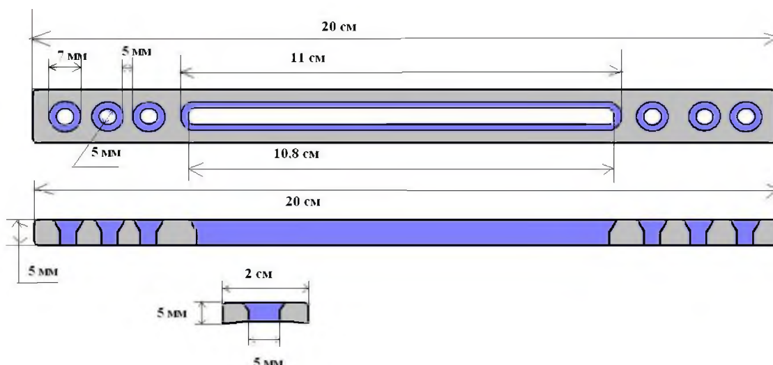
Рис. 1. Конструктивные особенности наkostной пластины.
